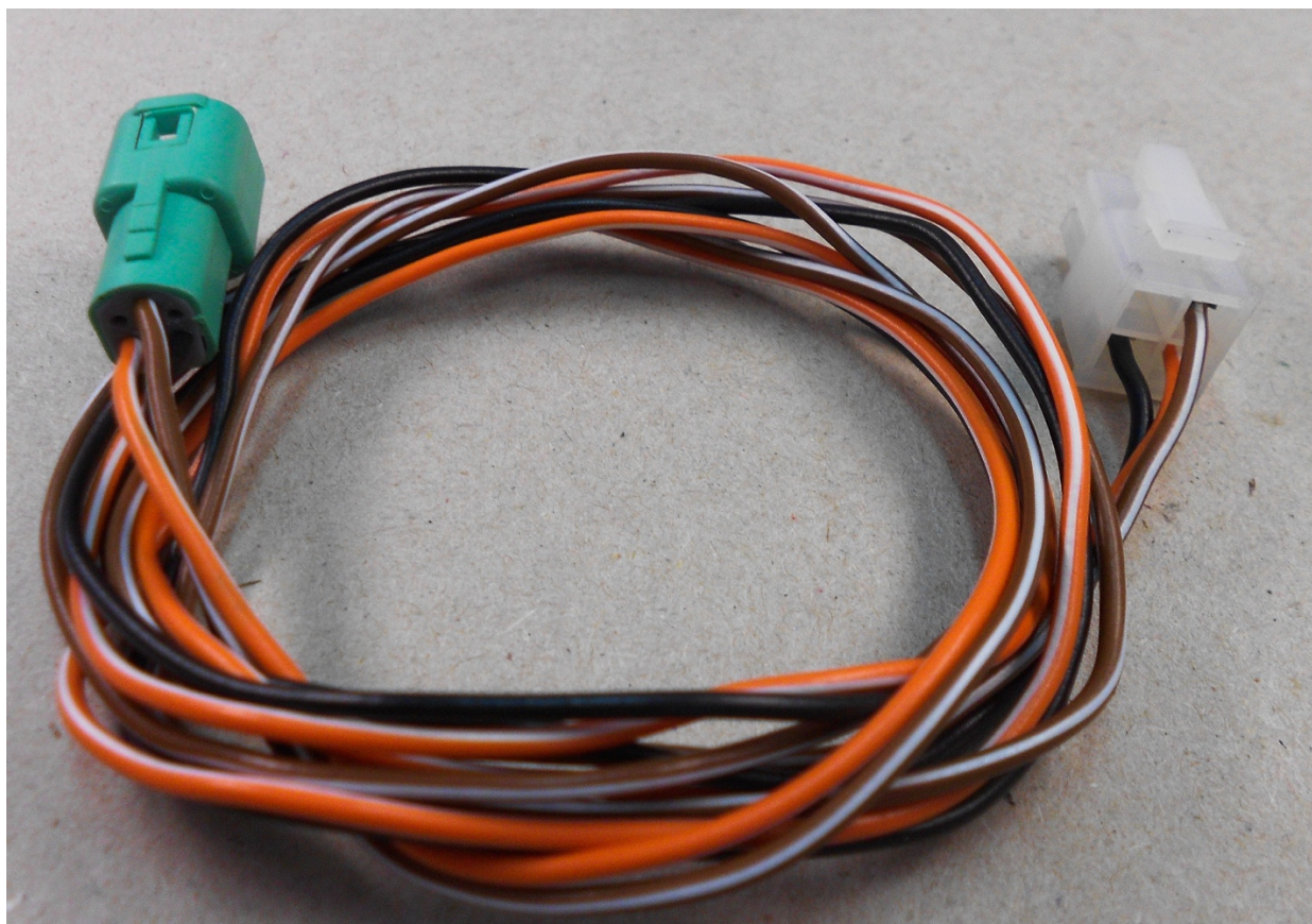
Общий вид кабеля в сборе
